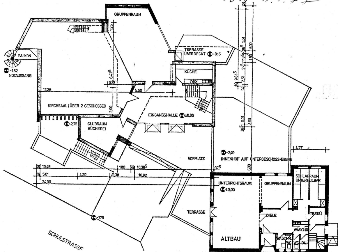
Abbildung 4: Grundriß des Gemeindeforums
